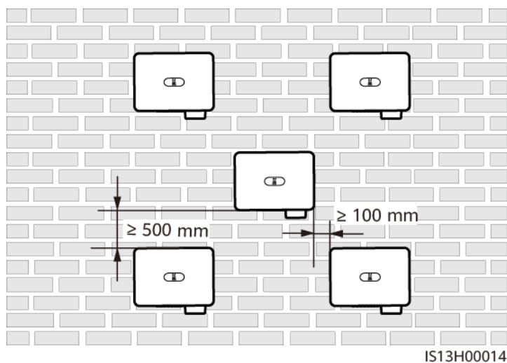
Rysunek 4-5 Trzypoziomowy montaż w układzie trójkąta (niezalecany)
