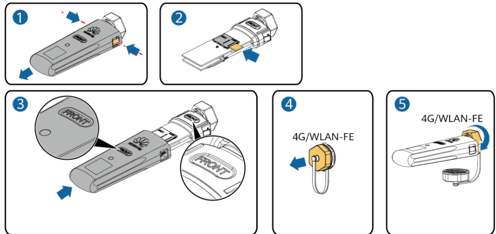
Rysunek 5-9 Montaż 4G Smart Dongle'a
