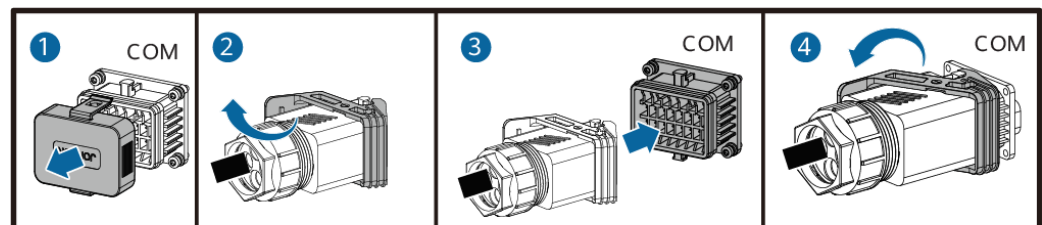
Rysunek 5-24 Mocowanie złącza sygnałowego
