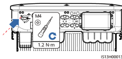
Rysunek 4-13 Montaż śruby blokującej do przetwornika DC
