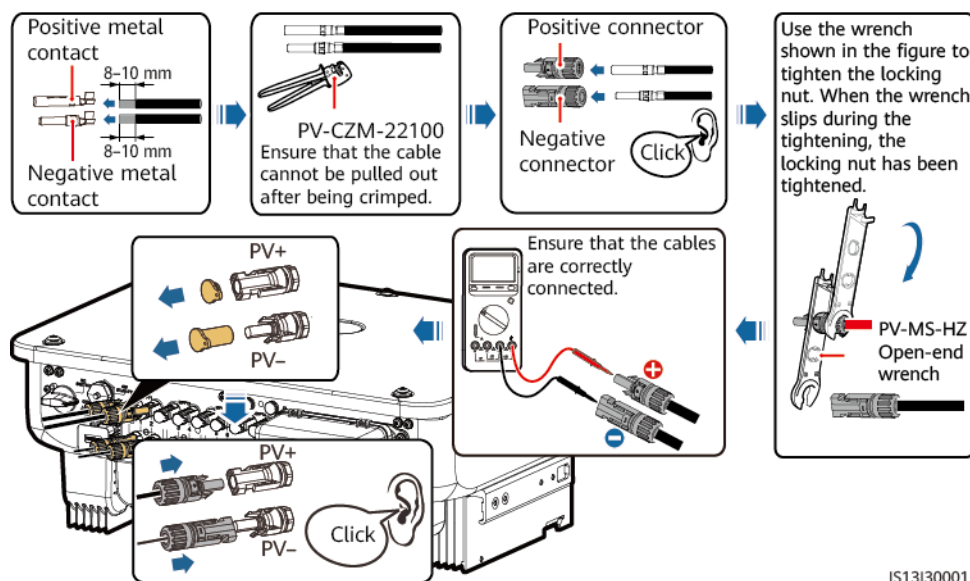
Rysunek 5-8 Podłączanie przewodu zasilającego DC
