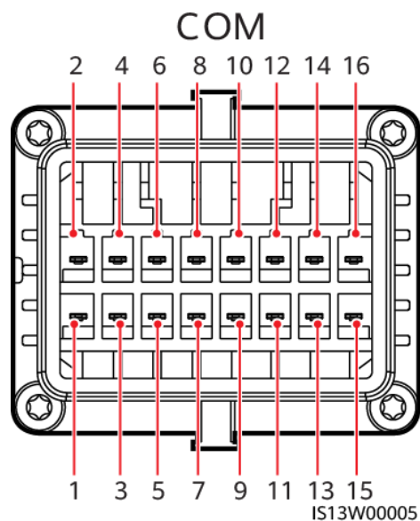
Rysunek 5-12 Oznaczenia pinów
