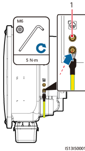
Rysunek 5-3 Podłączanie przewodu uziemiającego PE
