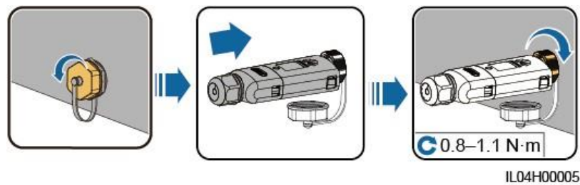
Rysunek 5-10 Montaż WLAN-FE Smart Dongle (komunikacja WLAN)
