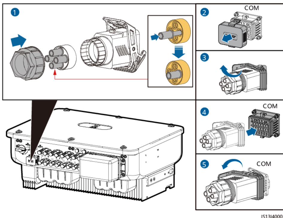
Rysunek 5-13 Mocowanie złącza sygnałowego
