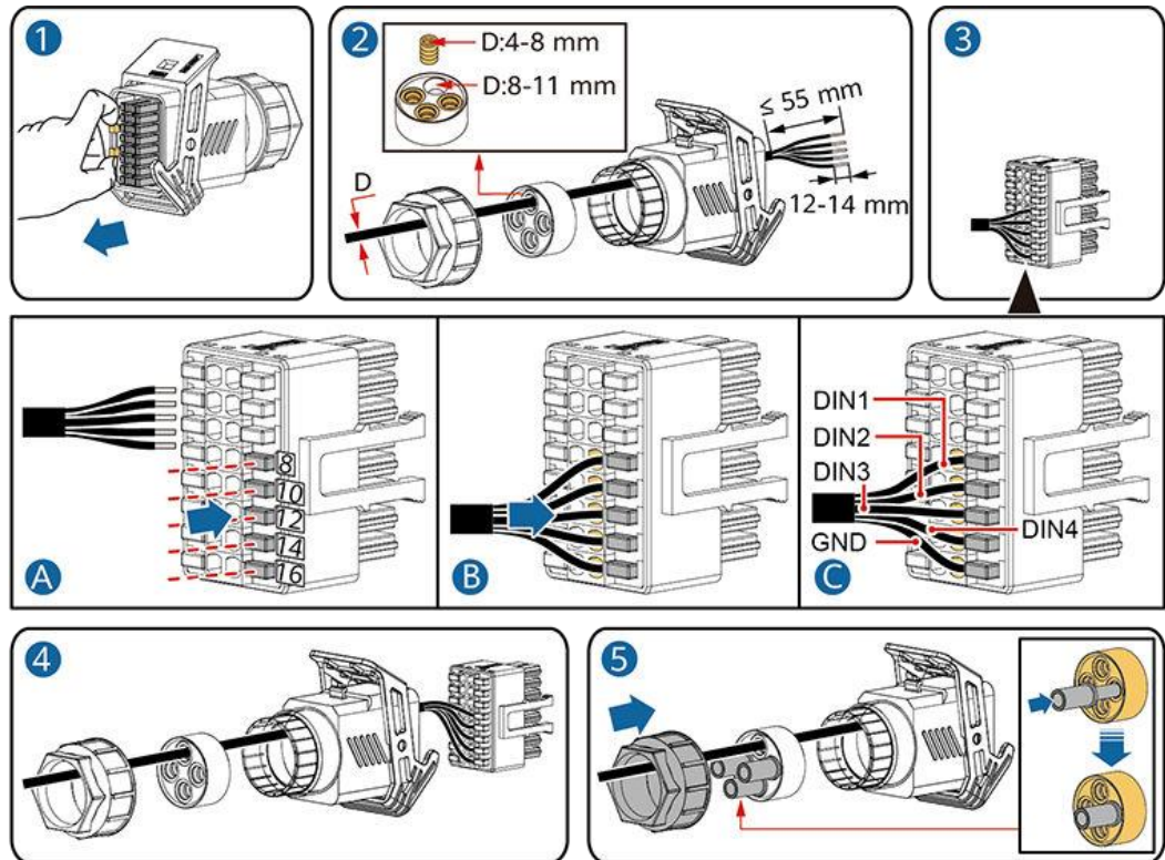
Rysunek 5-21 Podłączanie przewodu
