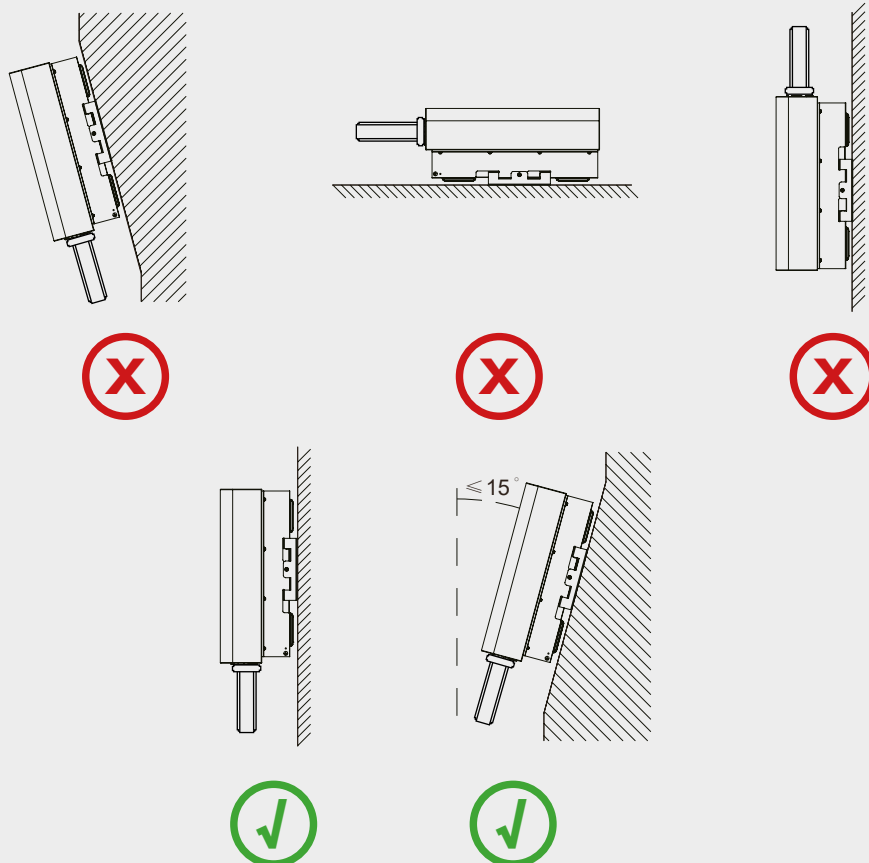
Kąt montażu Falownika
