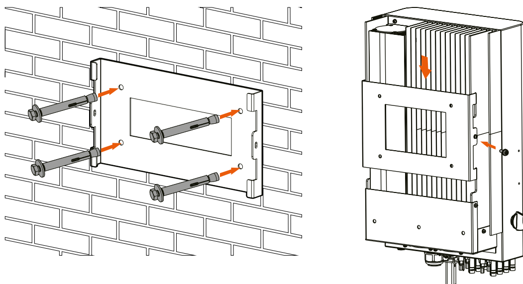
Instrukcja montażu ramy mocującej
