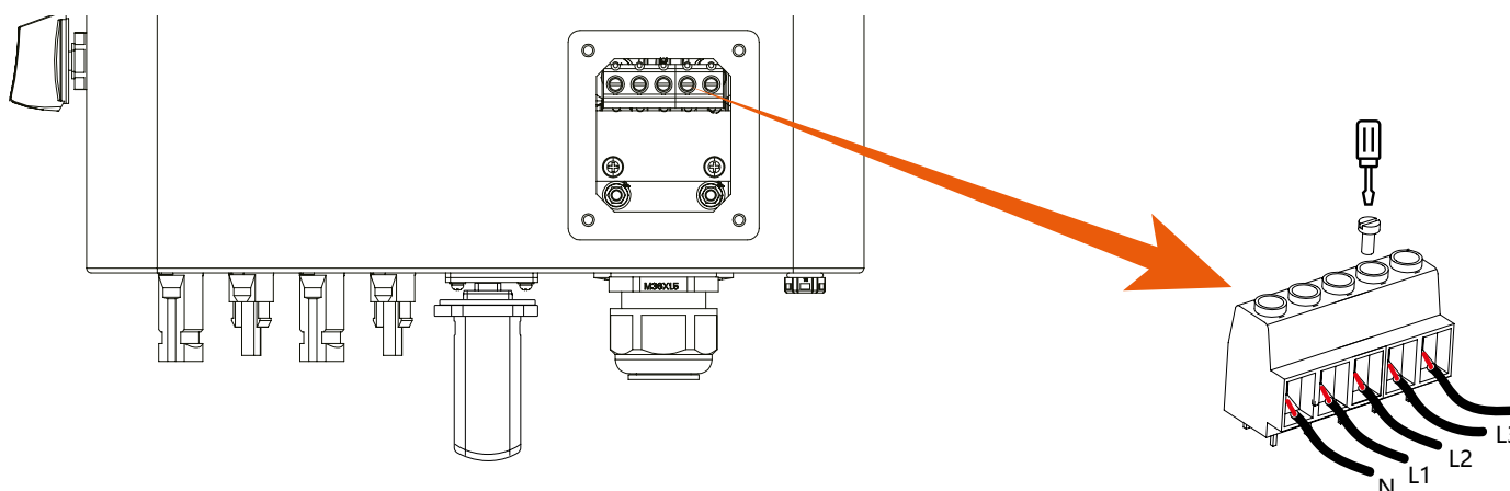
Schemat podłączenia AC
