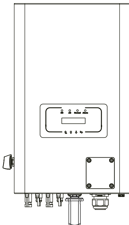
Przód Falownika
