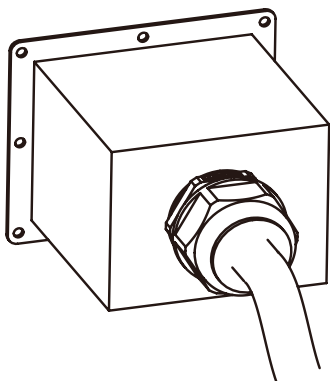
Przykład wprowadzonego przewodu poprzez pokrywę zabezpieczającą
