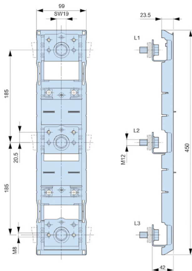
adapter DA 185-185/42
