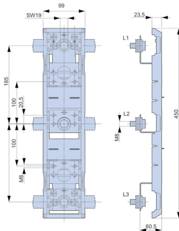
adapter DA 185-100/60
